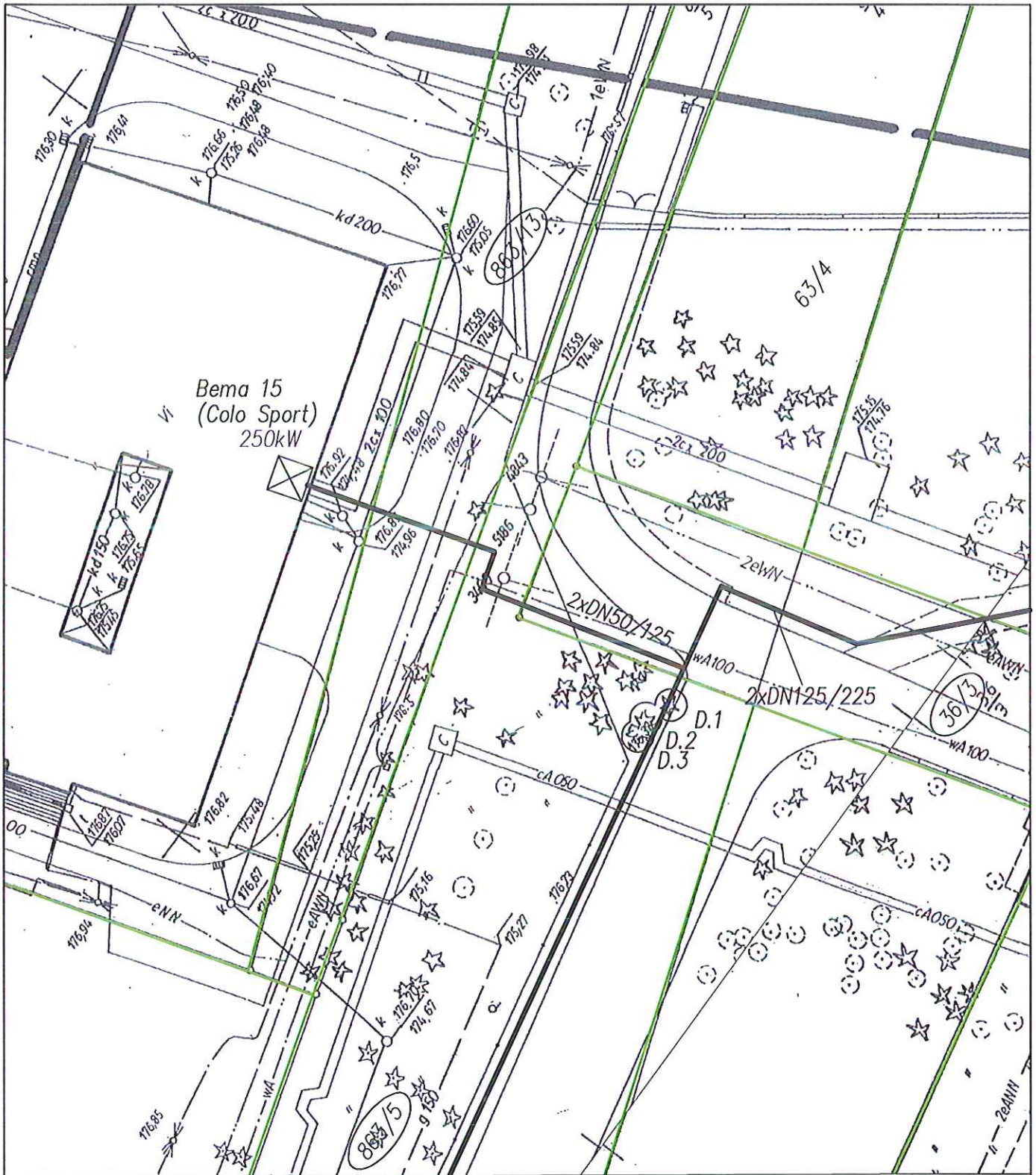
Projektowana sieć ciepłownicza
